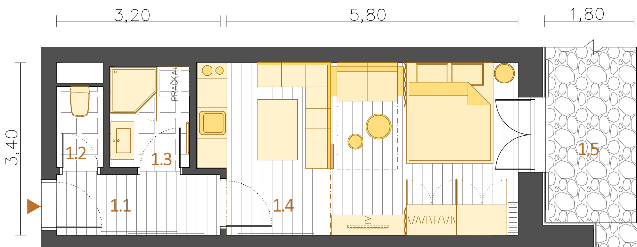
Půdorys bytu
