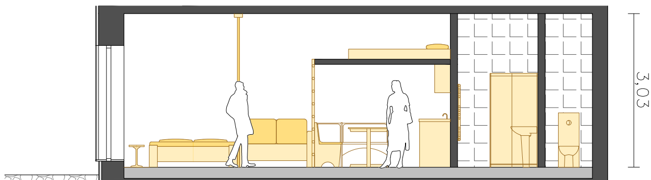
Řez bytem
