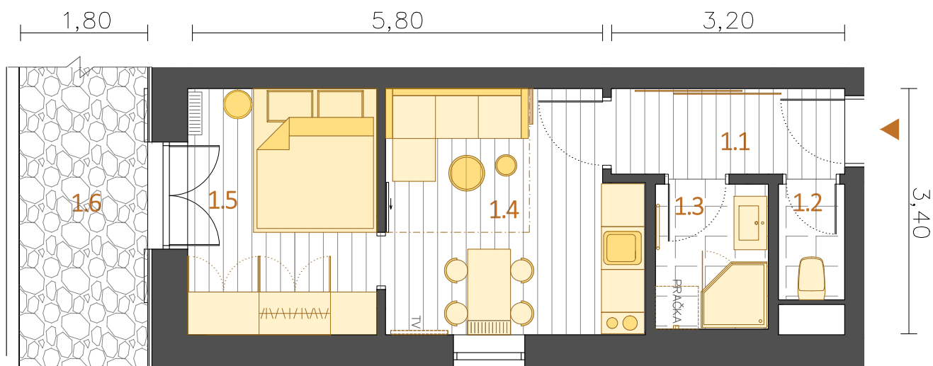
Půdorys bytu
