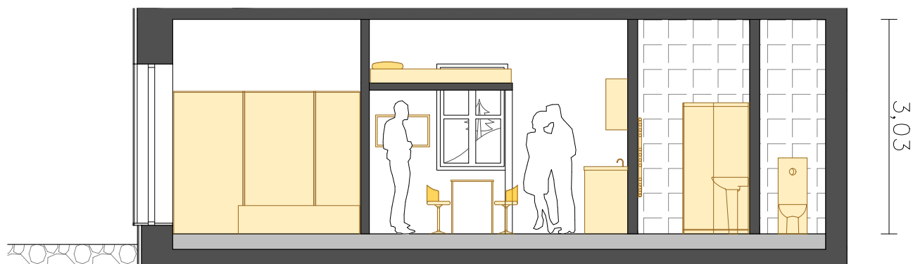
Řez bytem
