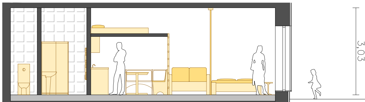
Řez bytem
